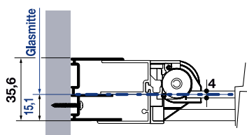
Position Wandprofil Tür
