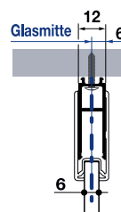
Position Wandprofil Seitenwand
