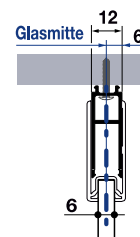
Position Wandprofil Seitenwand
