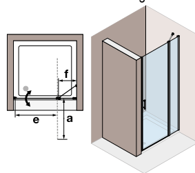
46 Art. 8U-4TN2 R Anschlag rechts
