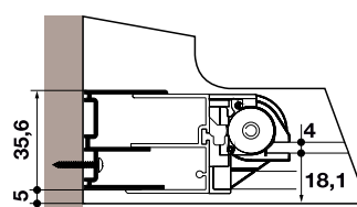
Position Wandprofil Tür / Eckeinstieg
