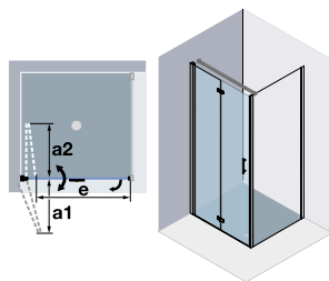
Art. 8U-4FPW L Anschlag links
