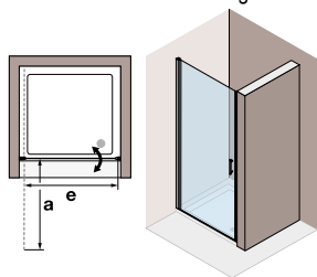
Art. 8U-4PTN1 L Anschlag links
