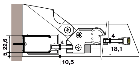
Position Wandprofil Tür
