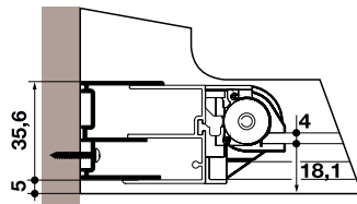
Position Wandprofil Tür
