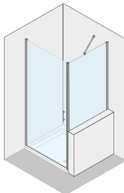
Art. 8U-4FPN L/R mit 8U-6SV L/R
