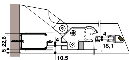
Position Wandprofil Tür / Eckeinstieg
