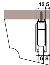
Position Wandprofil Seitenwand
