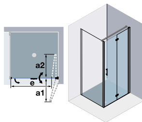
Art. 8U-4FPW R Anschlag rechts
