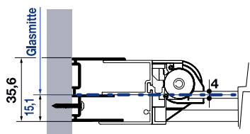
Position Wandprofil Tür
