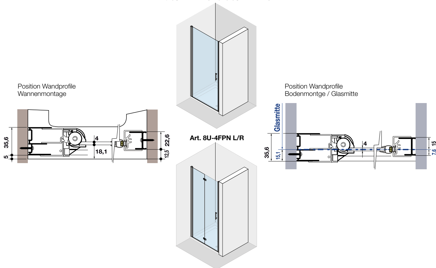
Art. 8U-4PTN1 L/R und 8U-4BPT1 L/R
