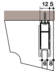
Position Wandprofil Seitenwand
