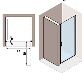
Art. 8U-4PTN1 R Anschlag rechts
