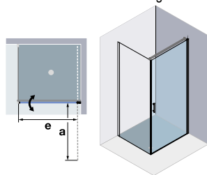
Art. 8U-4PTW1 R Anschlag rechts
